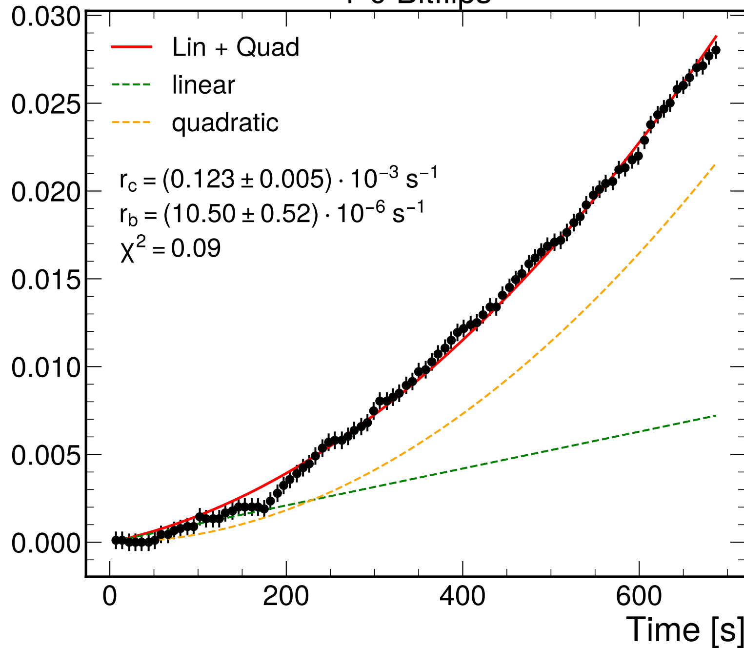
1-0 Bitflips
