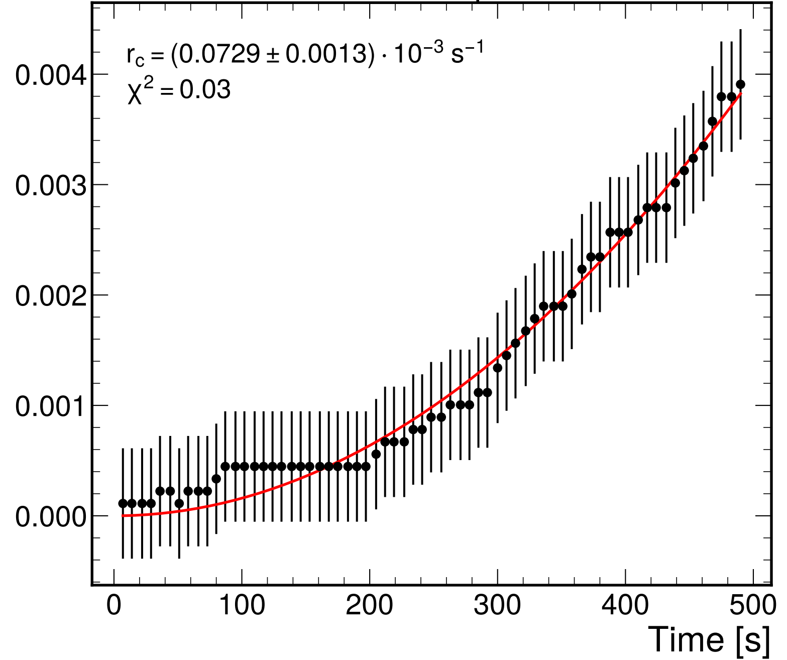
1-0 Bitflips
