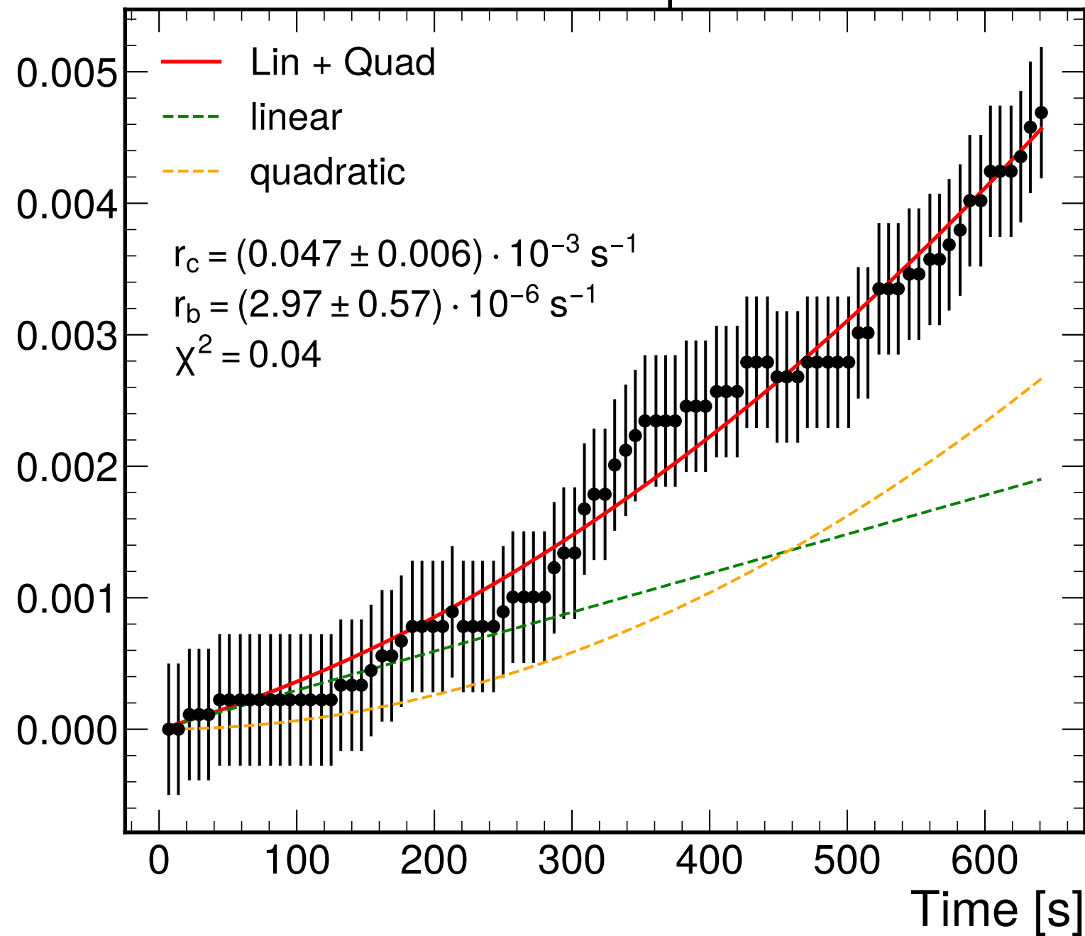
1-0 Bitflips
