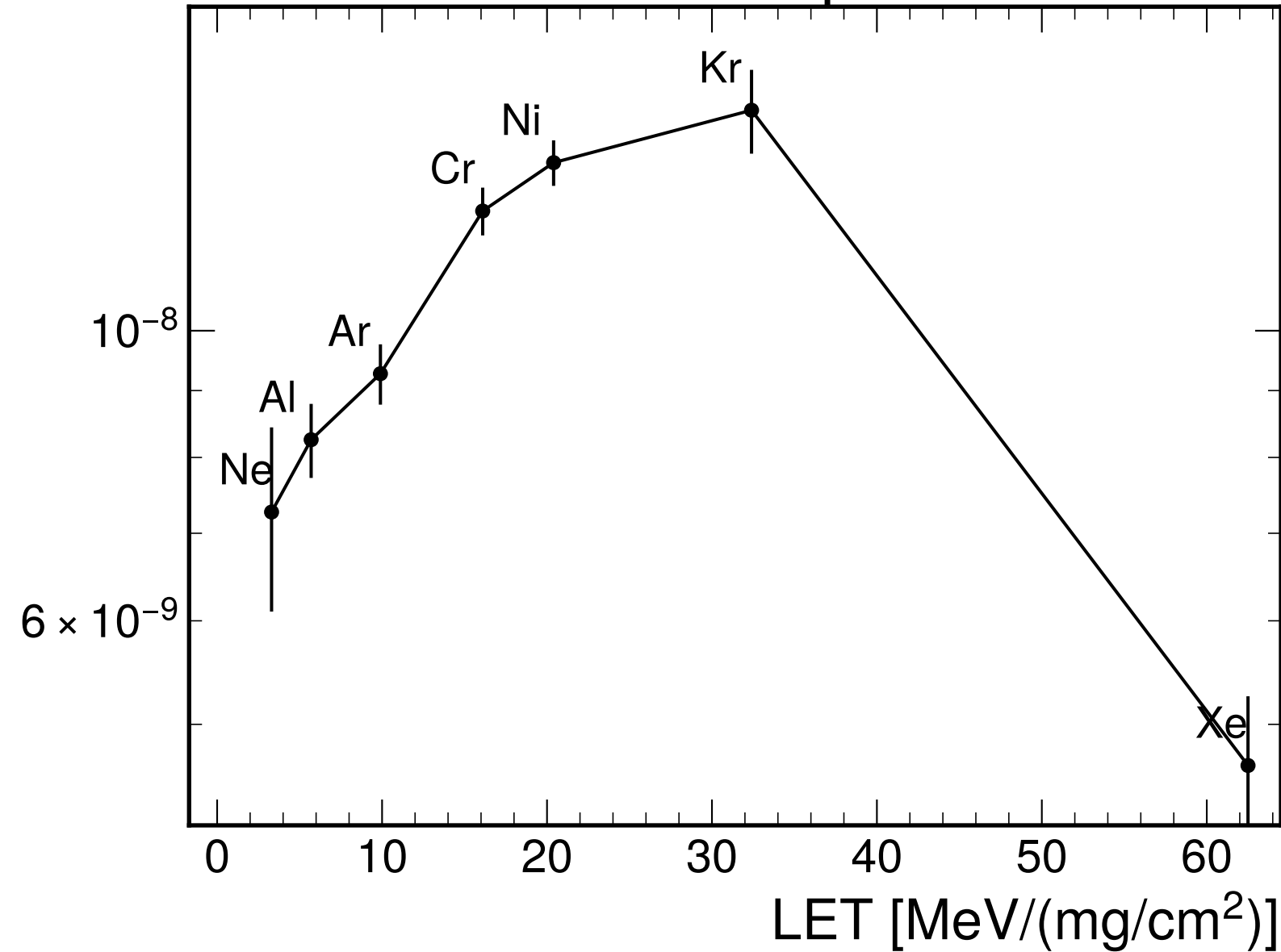
1-0 Bitflips
