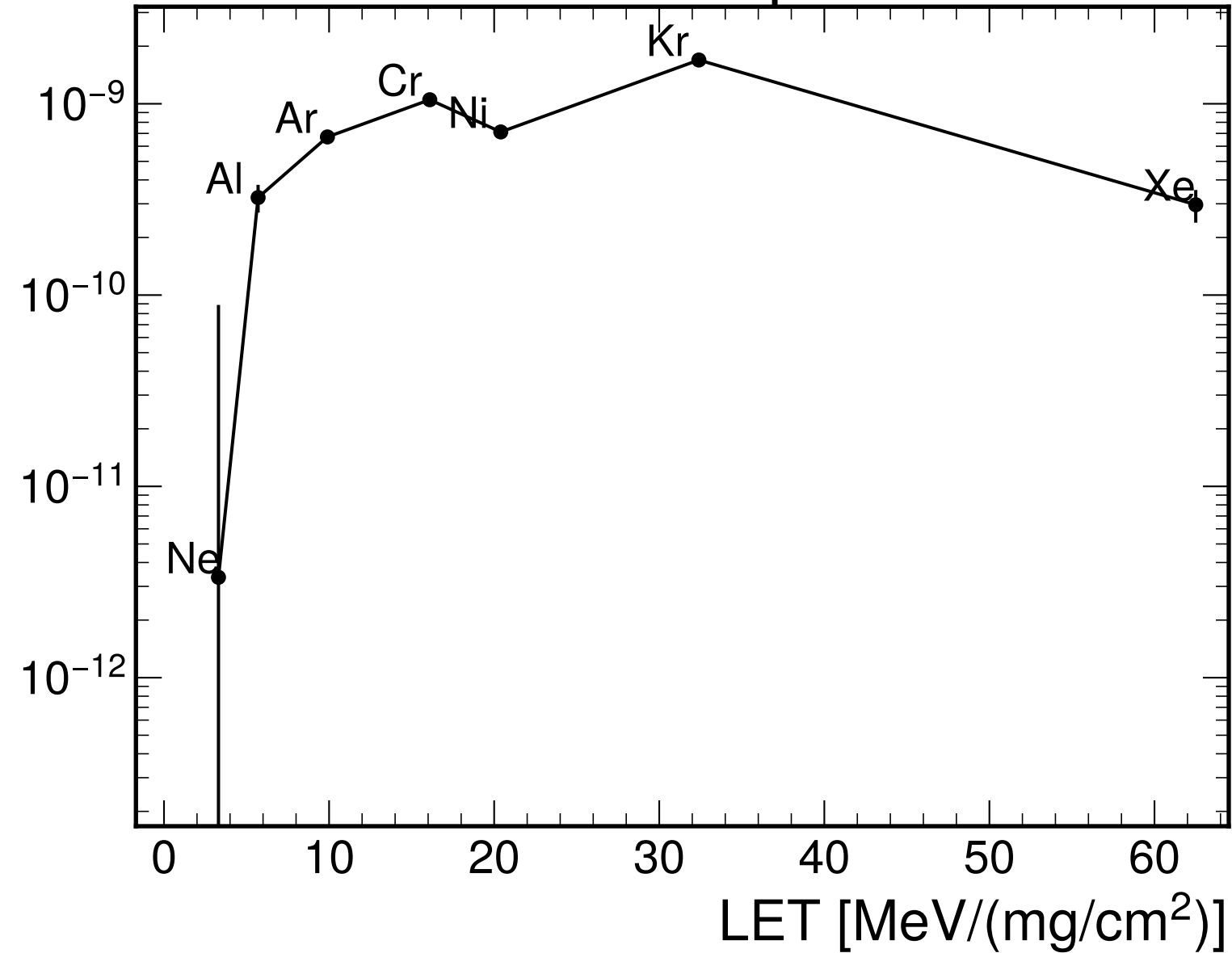
1-0 Bitflips
