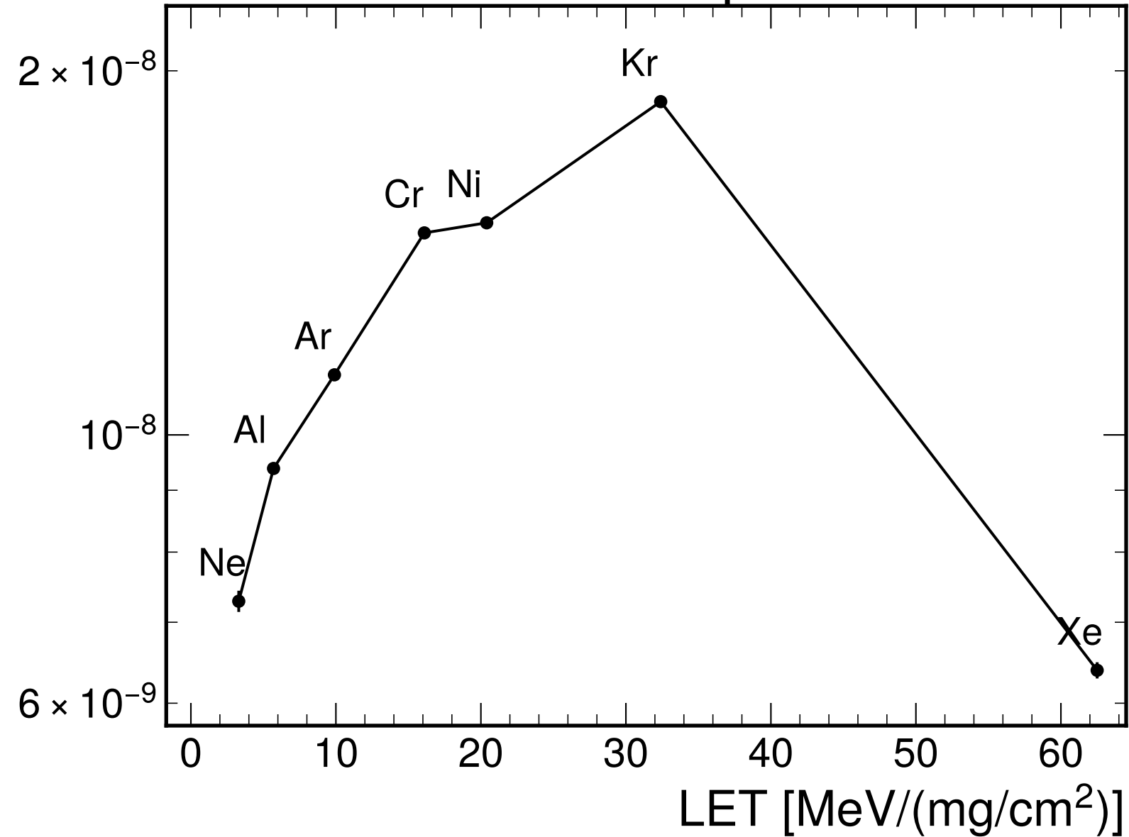
1-0 Bitflips
