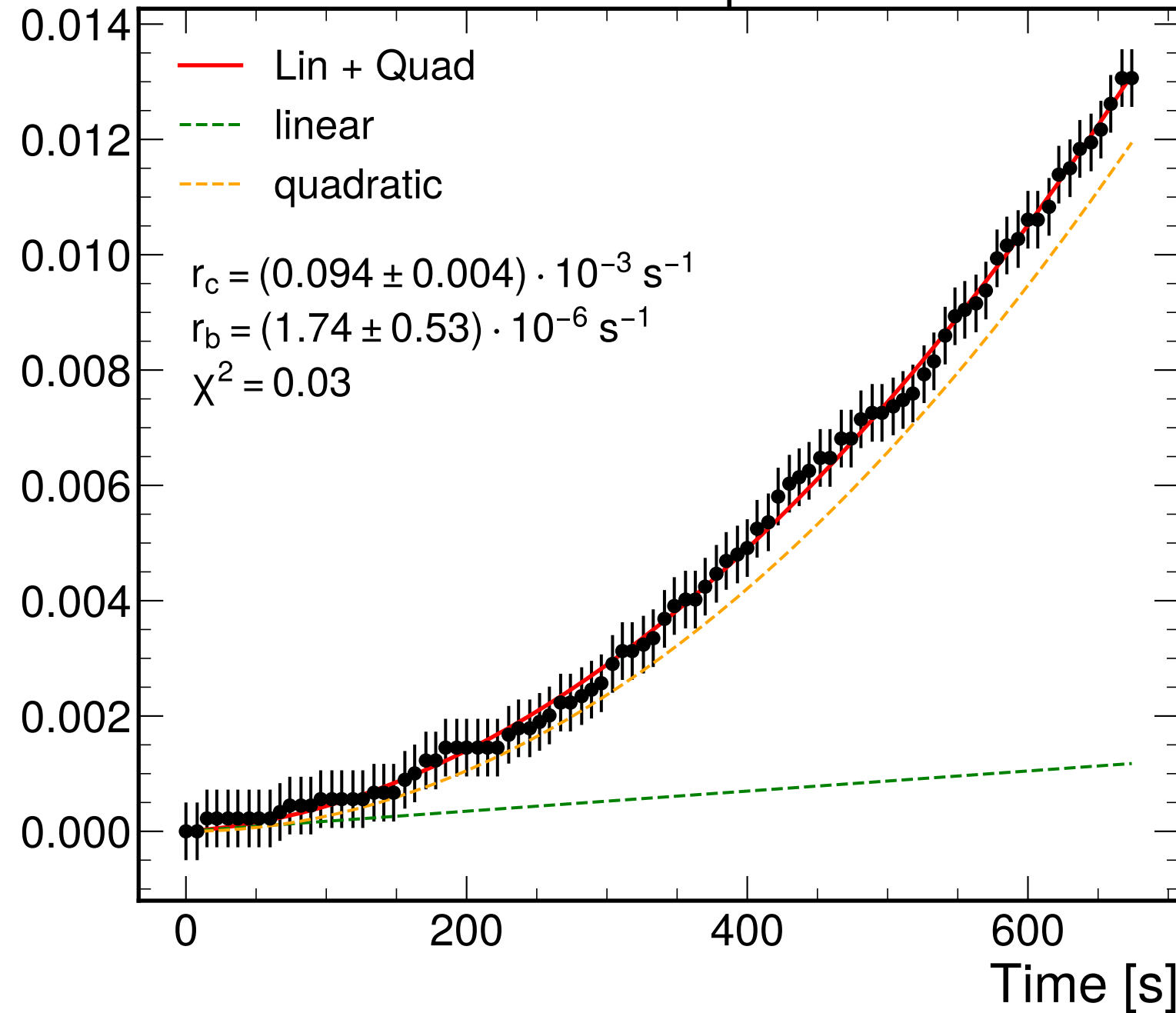
1-0 Bitflips
