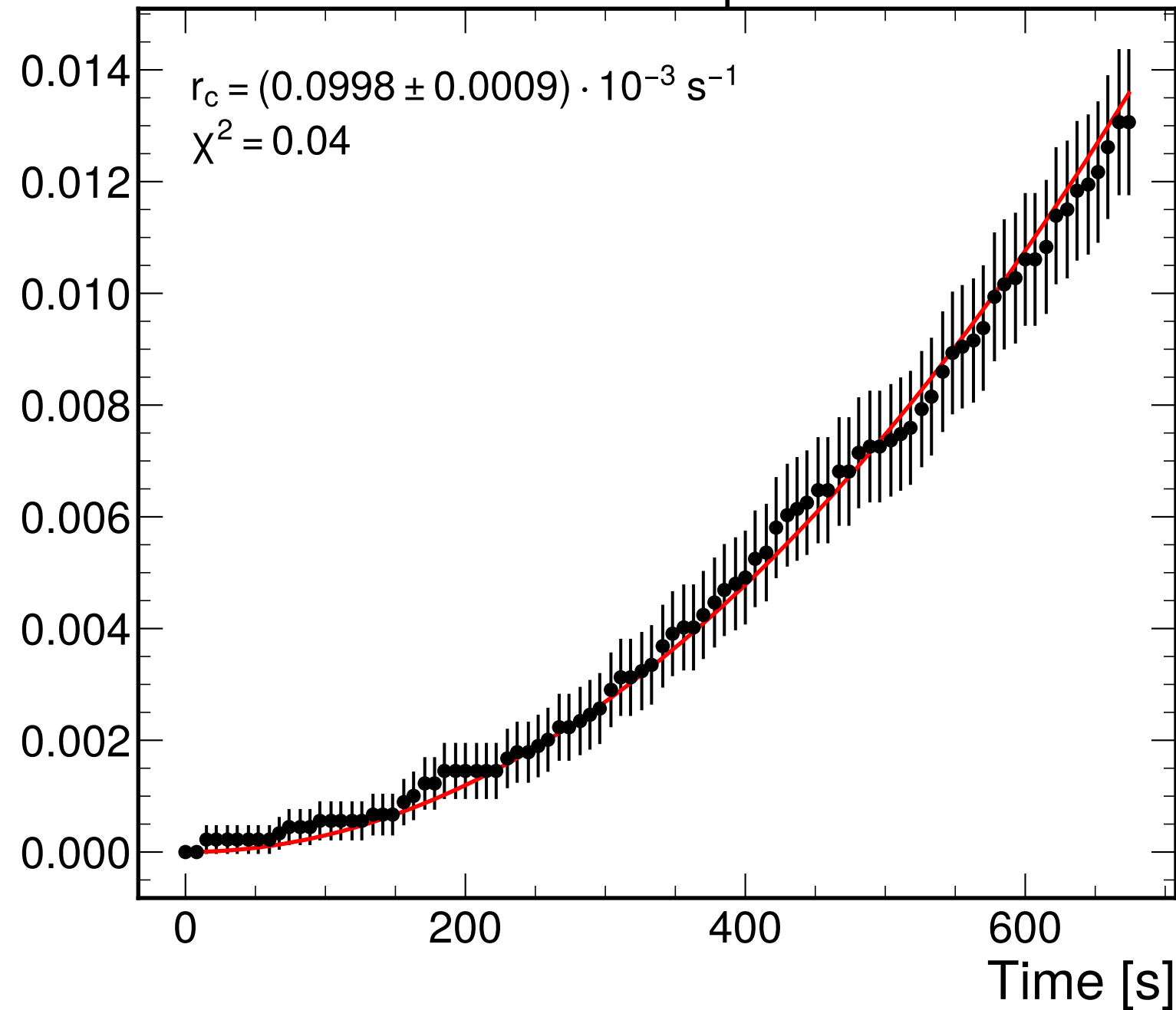
1-0 Bitflips
