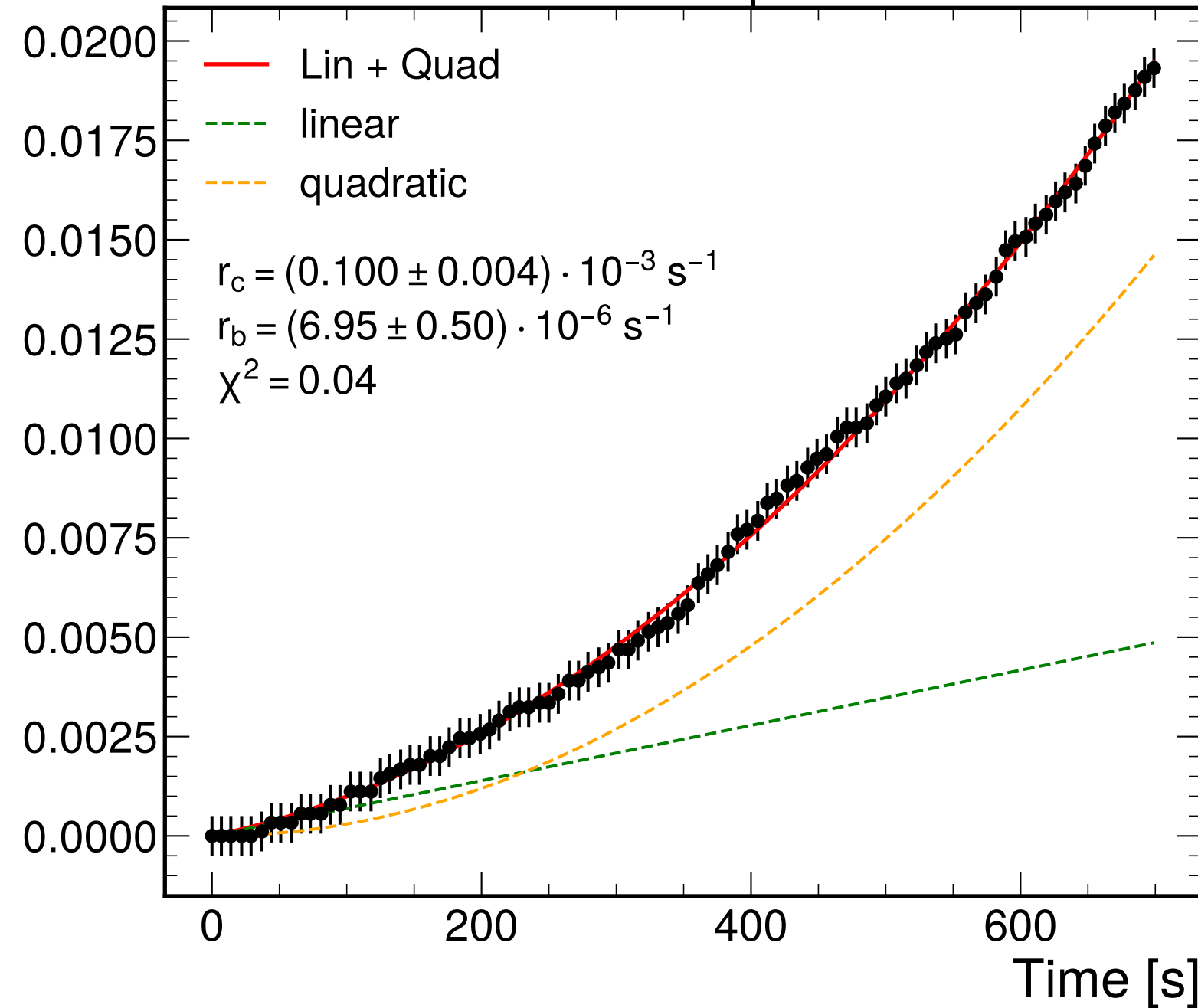
1-0 Bitflips
