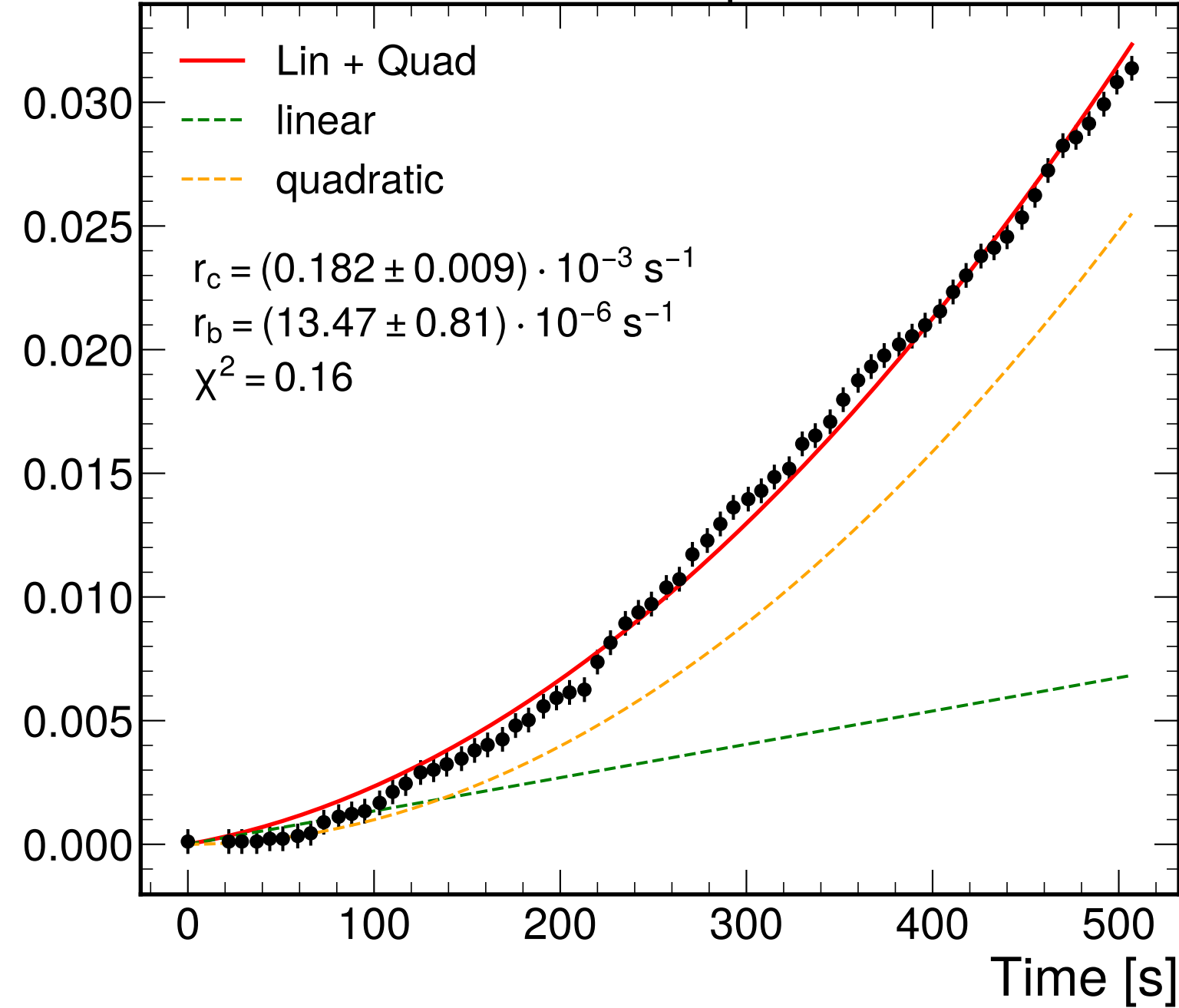
1-0 Bitflips
