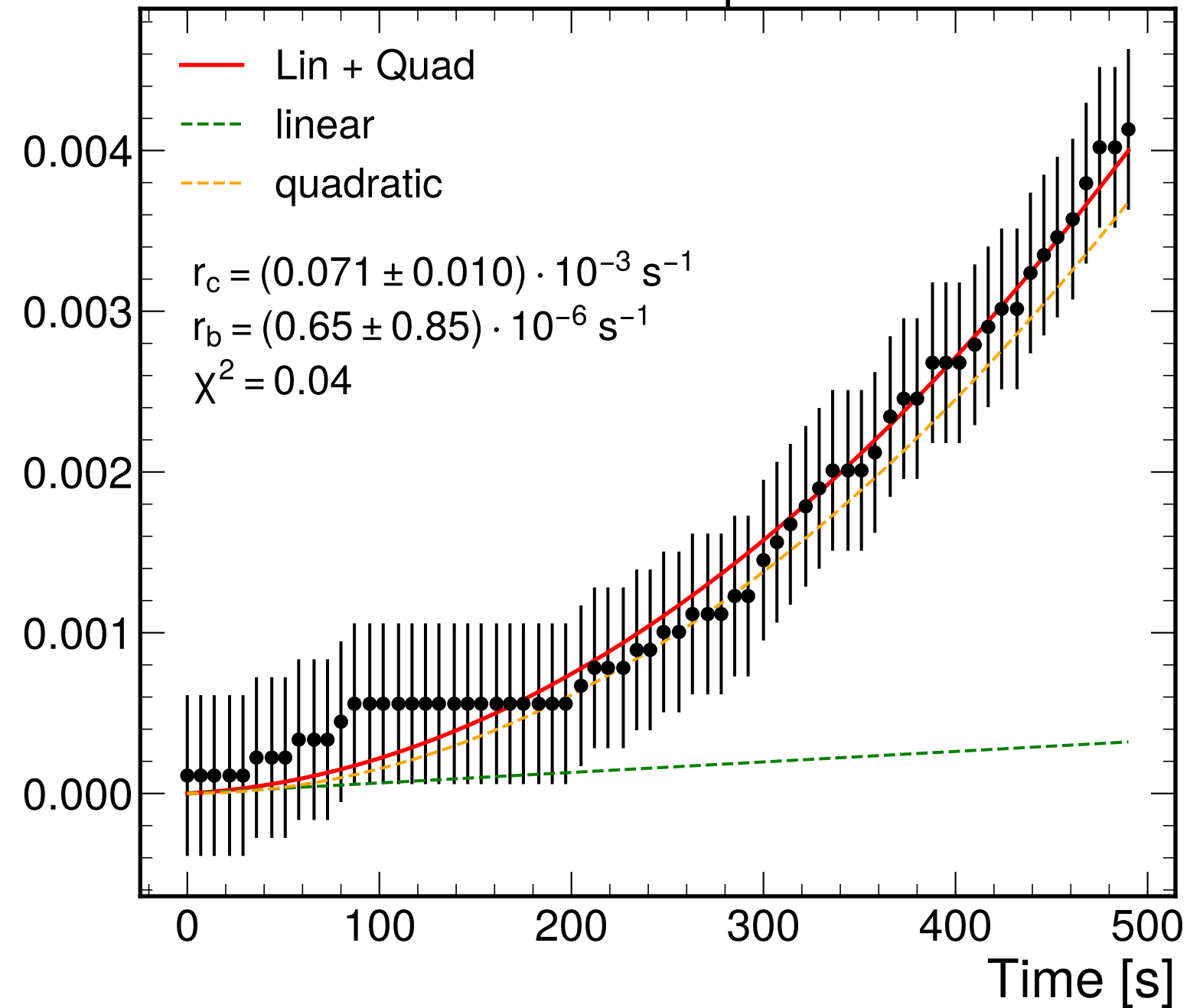
1-0 Bitflips
