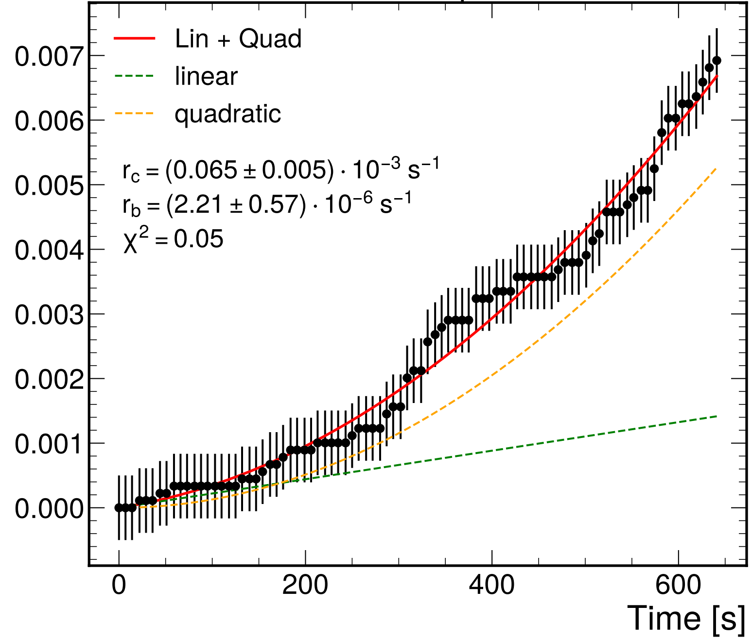
1-0 Bitflips
