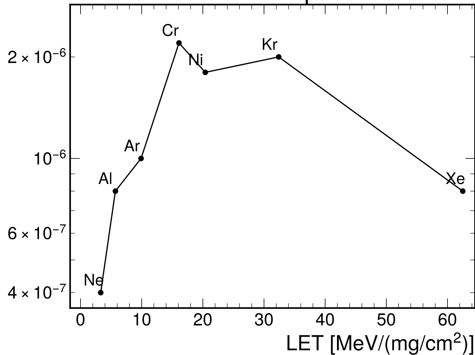
1-0 Bitflips
