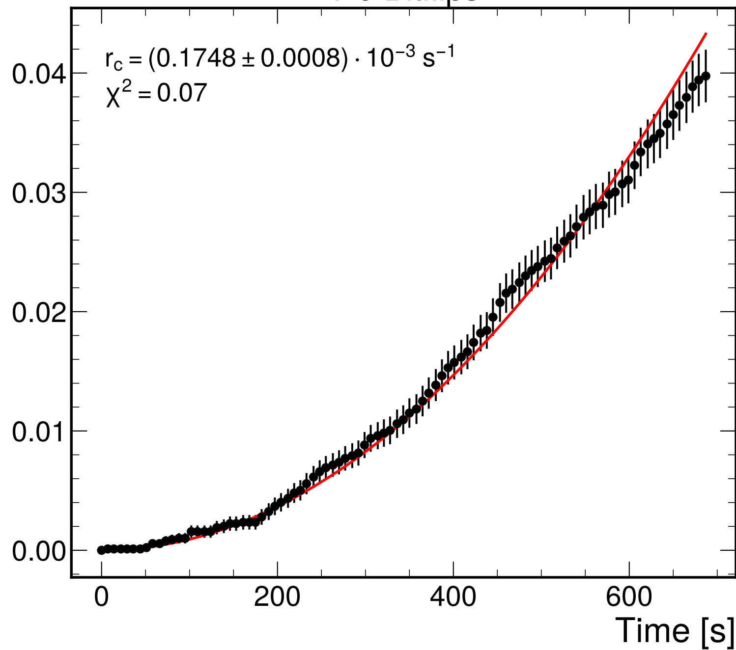
1-0 Bitflips
