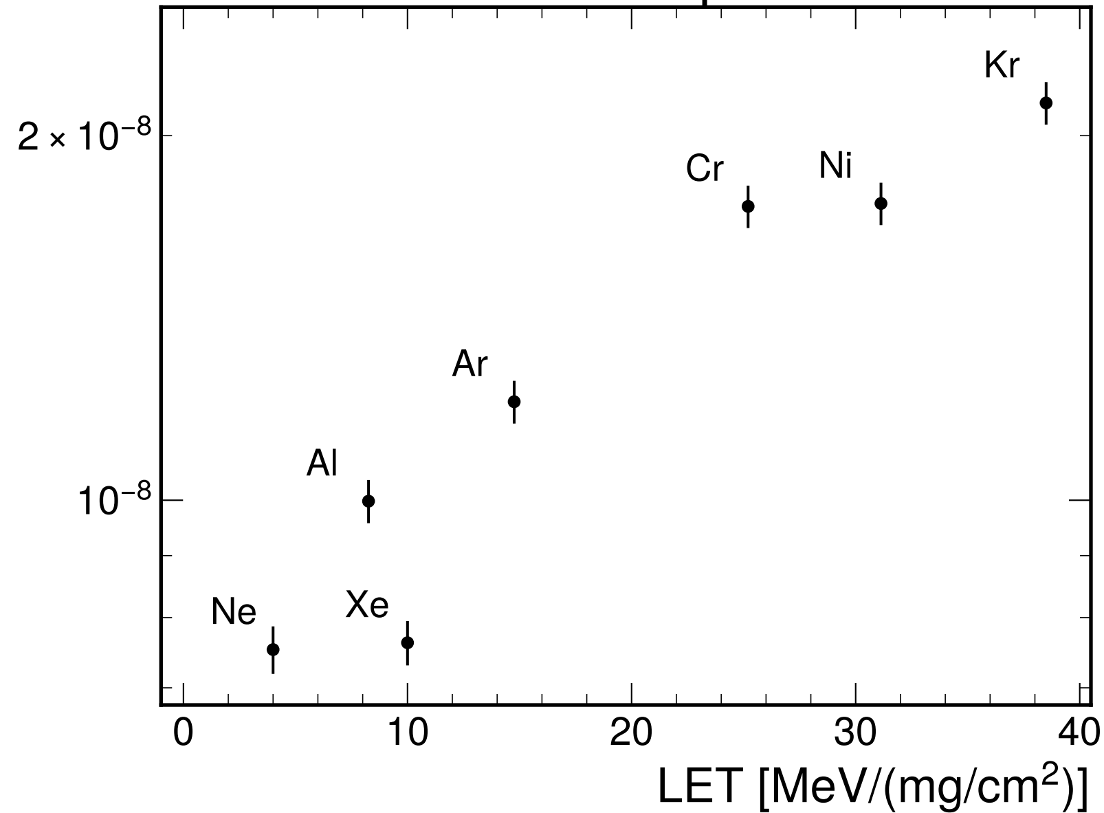
1-0 Bitflips
